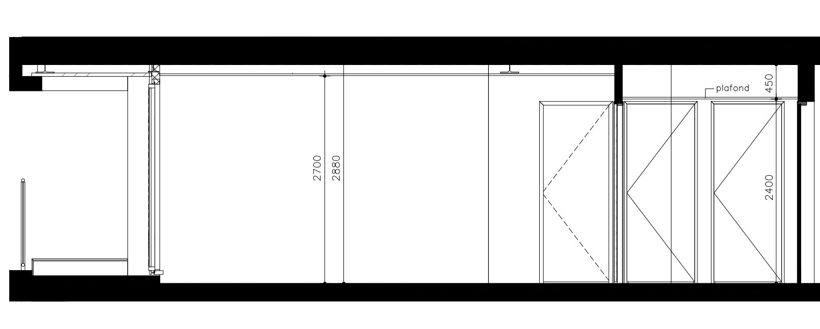
Doorsnede
